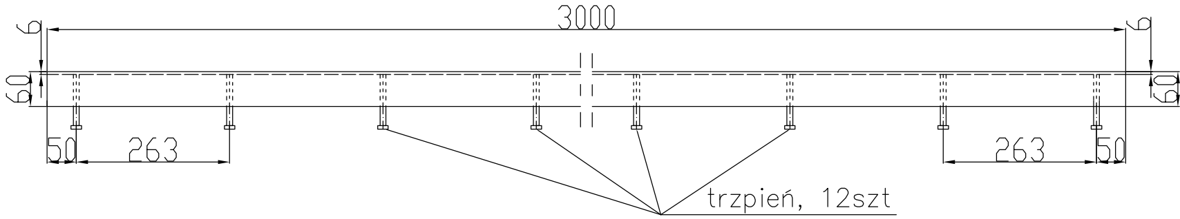
Rzut Skala 1:2
