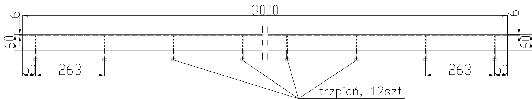
Rzut Skala 1:2
