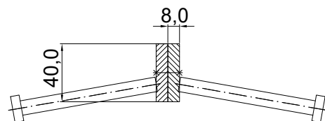
DOUBLE STRIP JOINT 08NA40 zbrojony Przekrój
