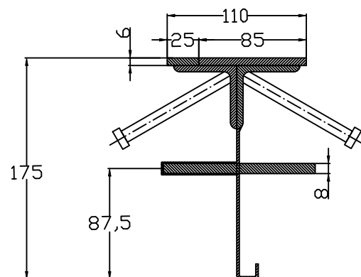
CONECTO 06NE110-5D-T8 h=175 Przekrój
