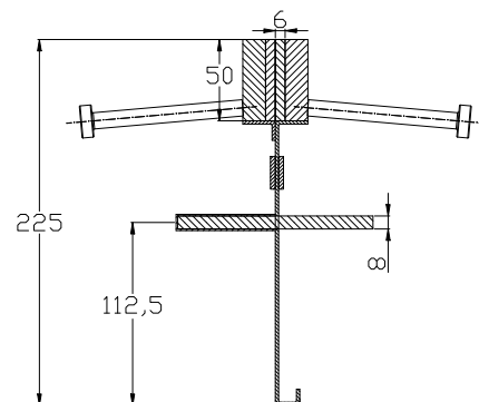
CONECTO SINUS 06NS50-4D-T8 h=225 PRZEKRÓJ
