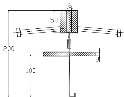
CONECTO SINUS 06NS50-4D-T8 h=200 Przekrój
