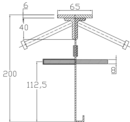
CONECTO SINUS 06NCC65/40x20-5D-T8 h=200 Przekrój
