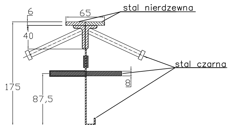
CONECTO SINUS 06NCC65/40x20-5D-T8 h=175 Przekrój
