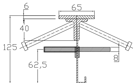
CONECTO SINUS 06NCC65/40x20-5D-T8 h=125 Przekrój
