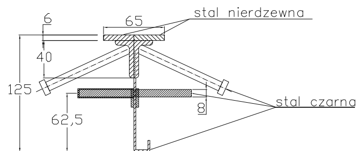
CONECTO SINUS 06NCC65/40x20-5D-T8 h=125 Przekrój
