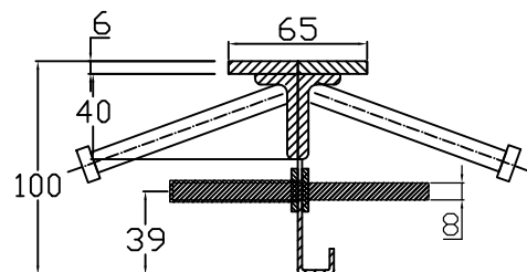
CONECTO SINUS 06NCC65/40x20-5D-T8 h=125 Przekrój
