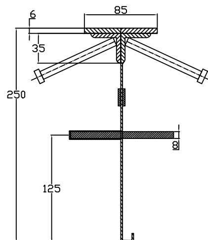
CONECTO SINUS 06NC85-5D-T8 h=250 Przekrój
