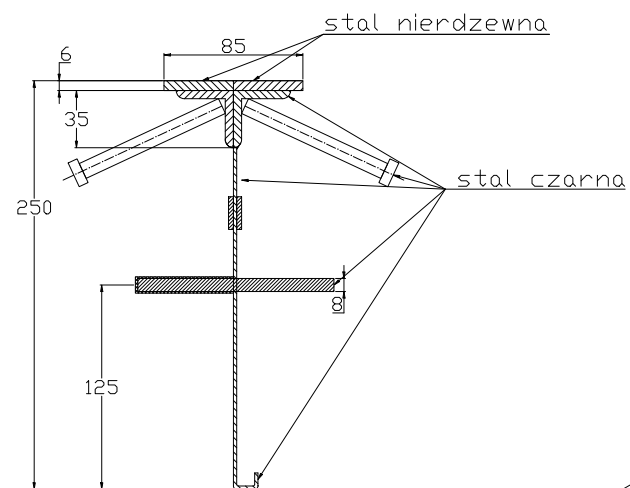
CONNECTO SINUS 06NC85-5D-T8 h=250 Przekrój
