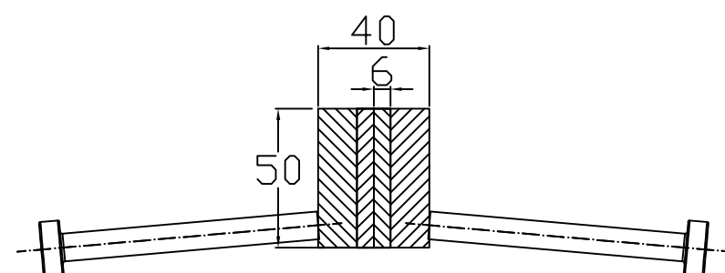
Conecto sinus 06NS50 zbrojony Przekrój
