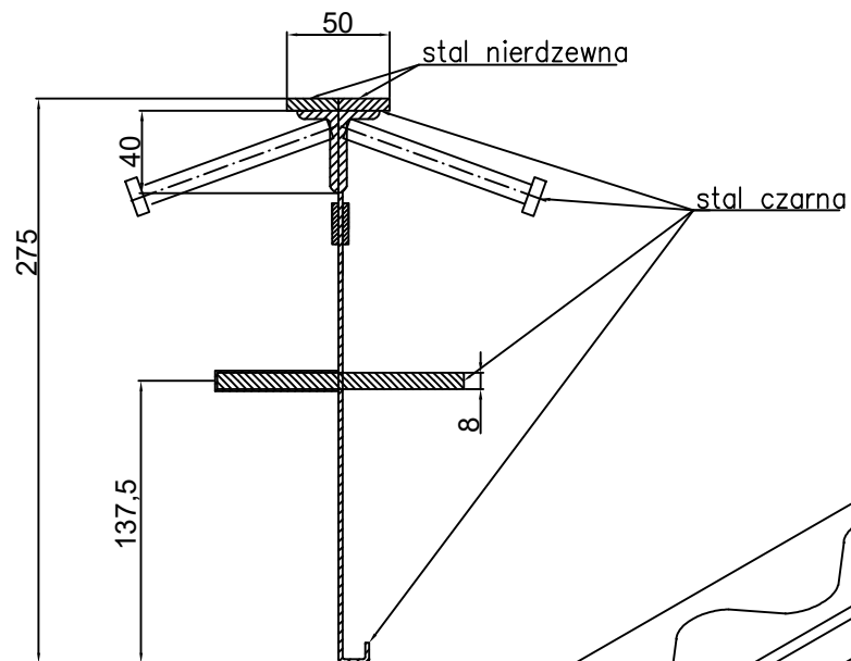
CONECTO SINUS 06NC50/20x40-5D-T8 h=275 Przekrój
