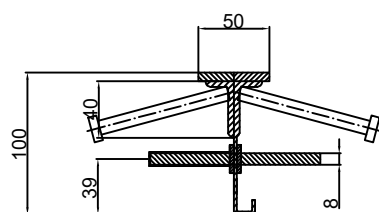
CONECTO SINUS 06NC50/20x40-5D-T8 h=100 Przekrój
