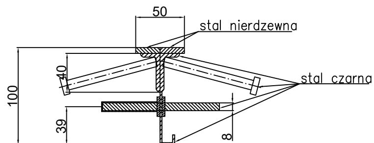
CONECTO SINUS 06NC50/20x40-5D-T8 h=100 Przekrój
