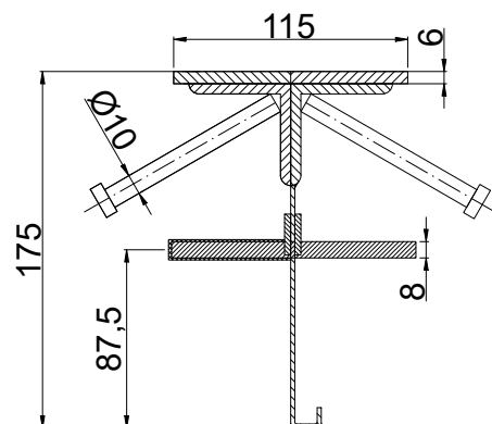
CONECTO SINUS 06NC115-5D-T8 h=175 Przekrój
