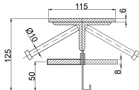
CONECTO SINUS 06NC115-5D-T8 h=125 Przekrój
