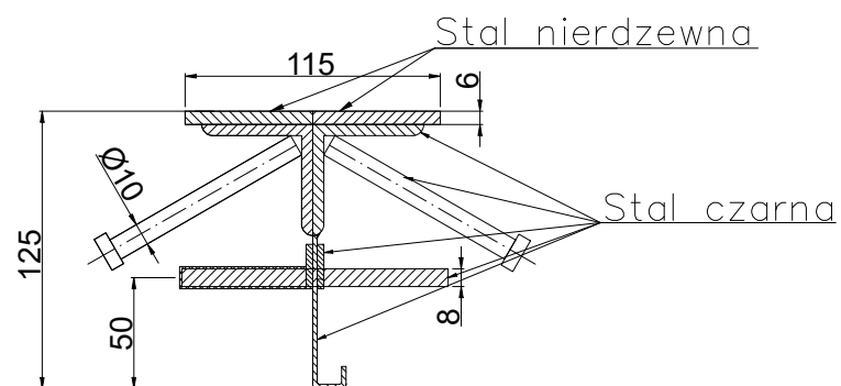
CONECTO SINUS 06NC115-5D-T8 h=125 Przekrój
