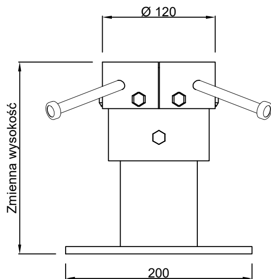
PRZEKRÓJ
