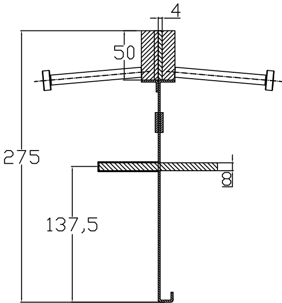
CONECTO SINUS 04NS50-4D-T8 h=275 Przekrój
