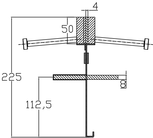
CONECTO SINUS 04NS50-4D-T8 h=225 Przekrój
