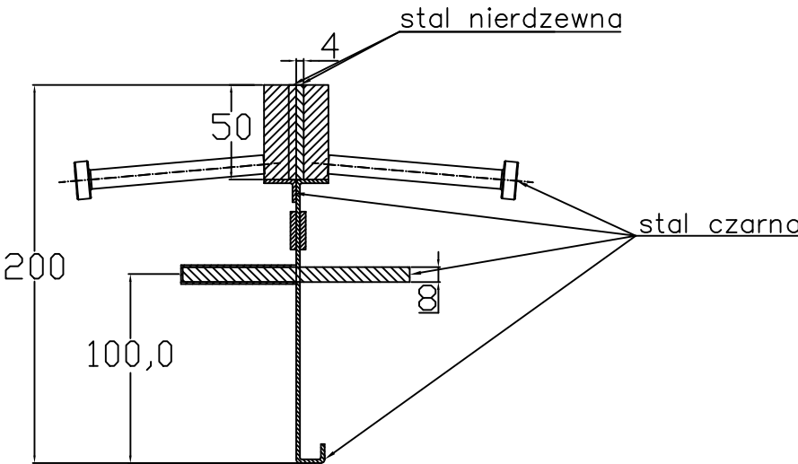
CONECTO SINUS 04NS50-4D-T8 h=200 Przekrój
