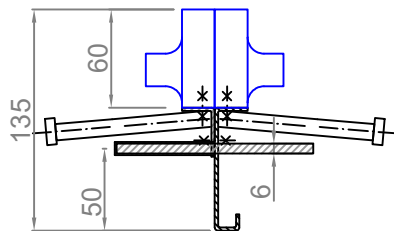
CONECTO SINUS 06NSTW60-5D-T6 h=135 Przekrój
