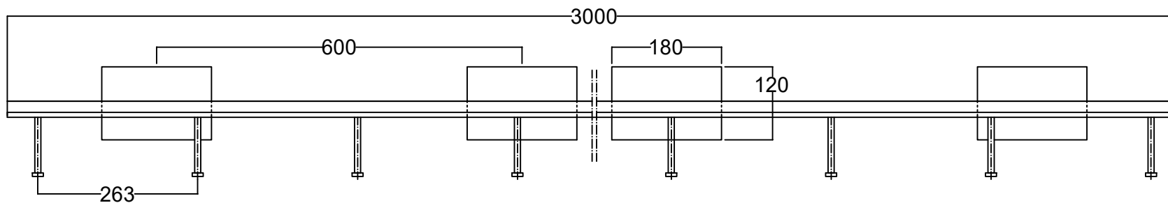
RZUT skala 1:1,25
