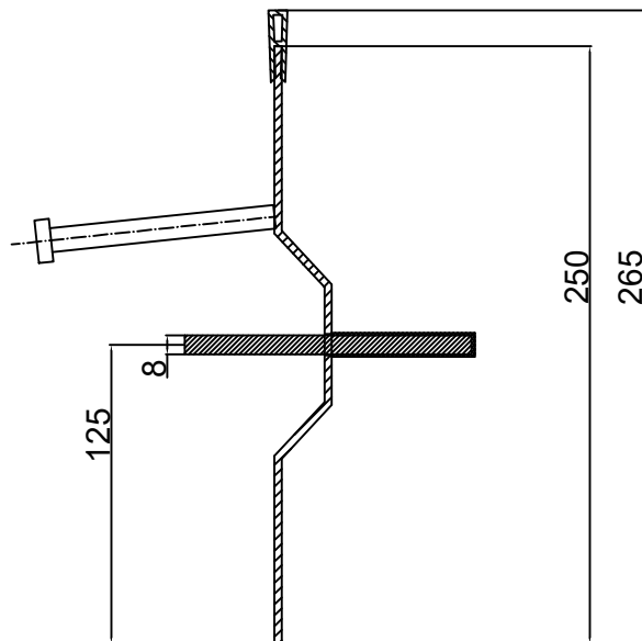
Profil dylatacyjny Omega 03NB-5D-T8 h=250/265
