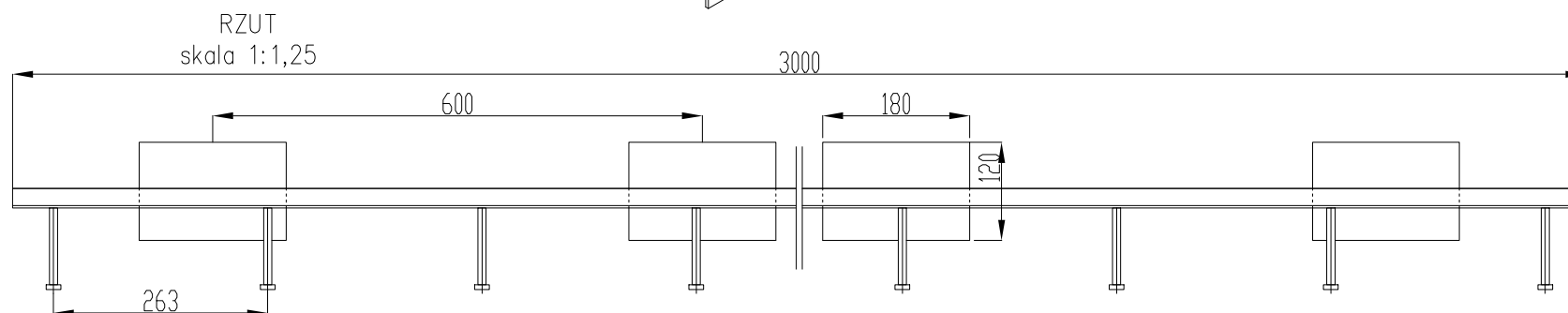
Profil dylatacyjny Omega 03NB-5D-T8 h=225/240
