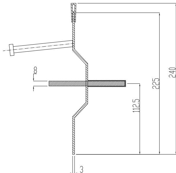
Profil dylatacyjny Omega 03NB-5D-T8 h=225/240
