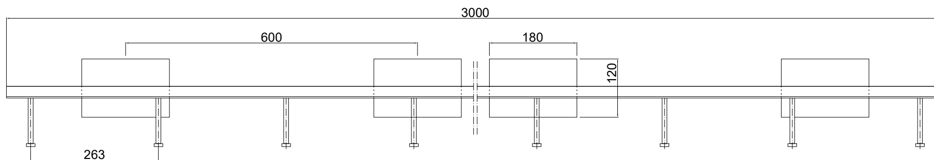
Omega 03NB-5D-T8 h=125 RZUT skala 1:1,25
