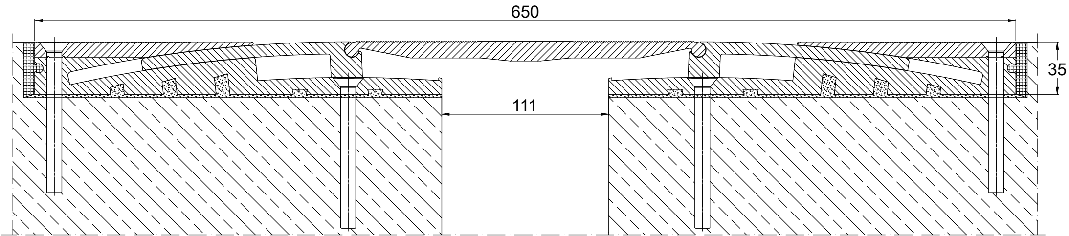
CONECTO HDS 650.100.35 PRZEKRÓJ
