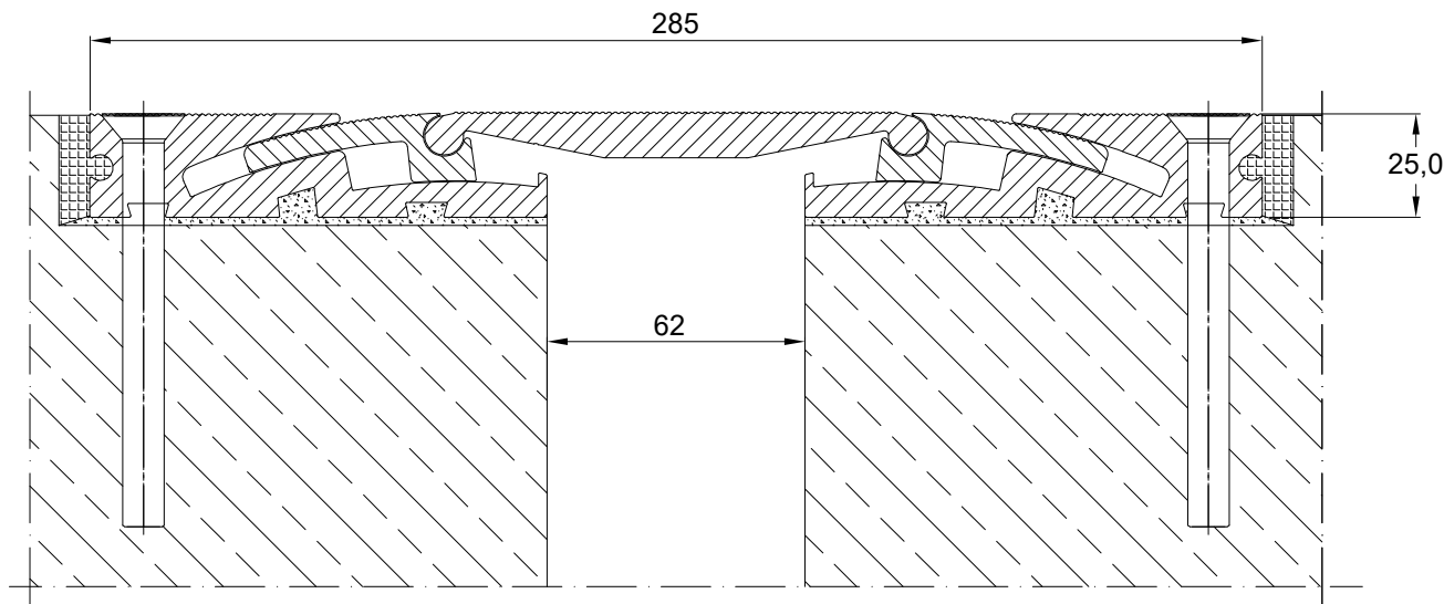
CONECTO HDS 285.30.25 PRZEKRÓJ
