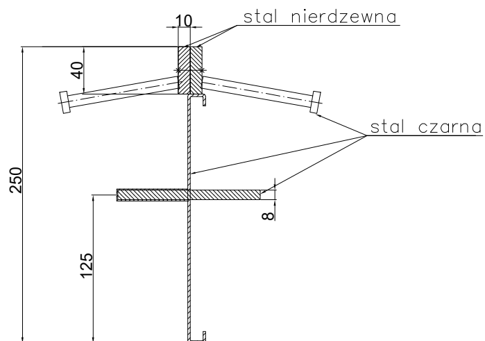
CONECTO DOWEL 10NA40-5D-T8 h=250 Przekrój
