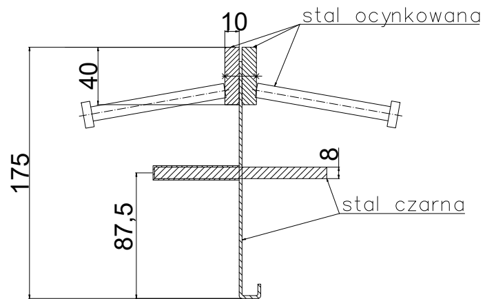
CONECTO DOWEL 10NA40-5D-T8 h=175 Przekrój Skala 2:1
