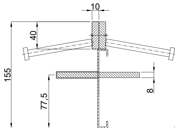
CONECTO DOWEL 10NA40-5D-T8 h=155 Prekrój Skala 2:1
