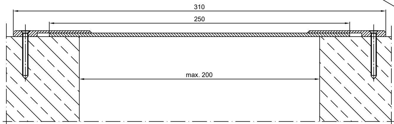
CONECTO WA 310 PRZEKRÓJ
