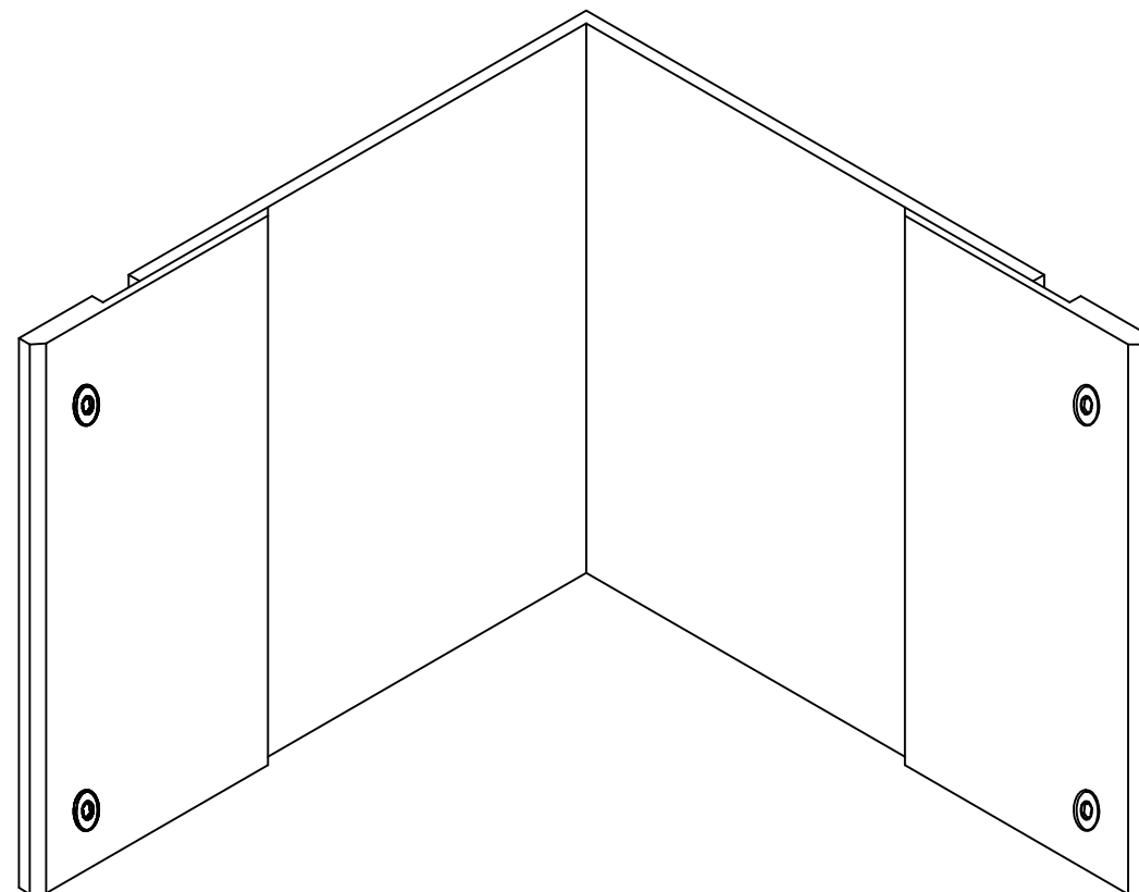
PROFIL DYLATACJNY WA 310 CV RZUT AKSONOMETRYCZNY
