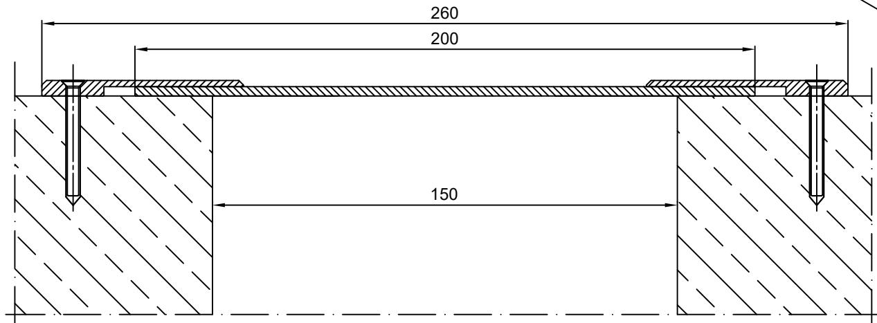
PROFIL DYLATACJNY WA 260 PRZEKRÓJ
