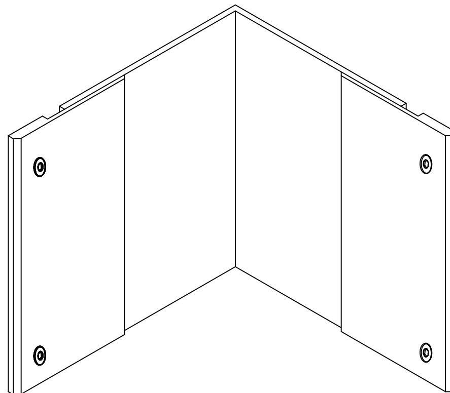
PROFIL DYLATACJNY WA 260 CV RZUT AKSONOMETRYCZNY
