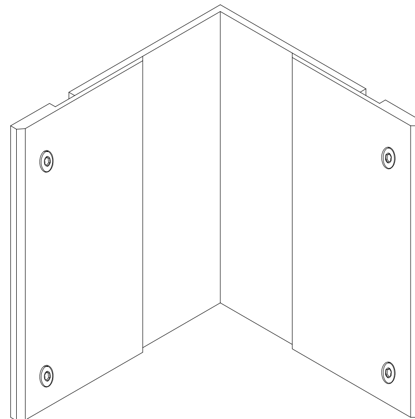
PROFIL DYLATACJNY WA 210 CV RZUT AKSONOMETRYCZNY
