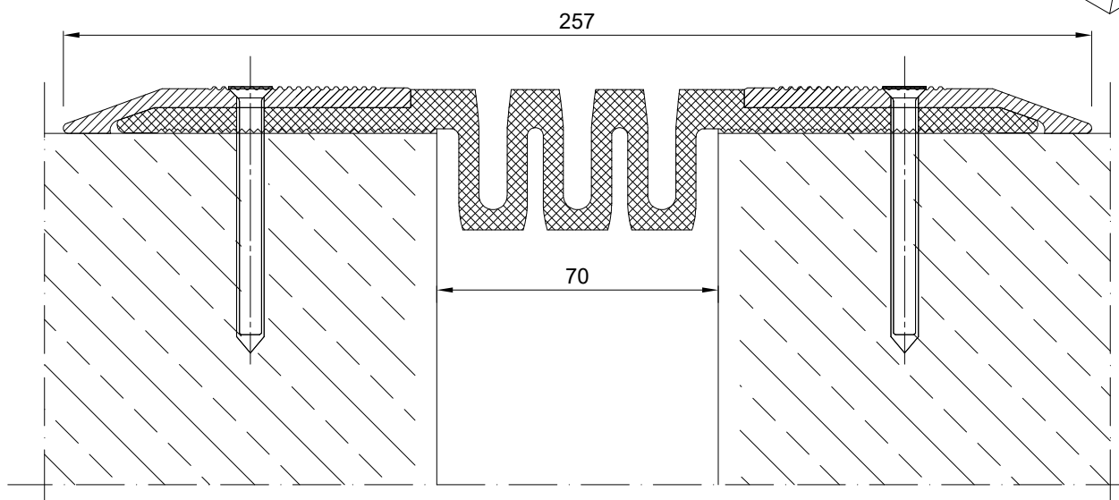
PROFIL DYLATAJNY SL 230.70.N PRZEKRÓJ
