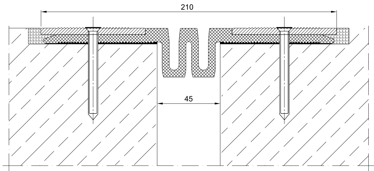
CONECTO PARK SL 210.50.W PRZEKRÓJ
