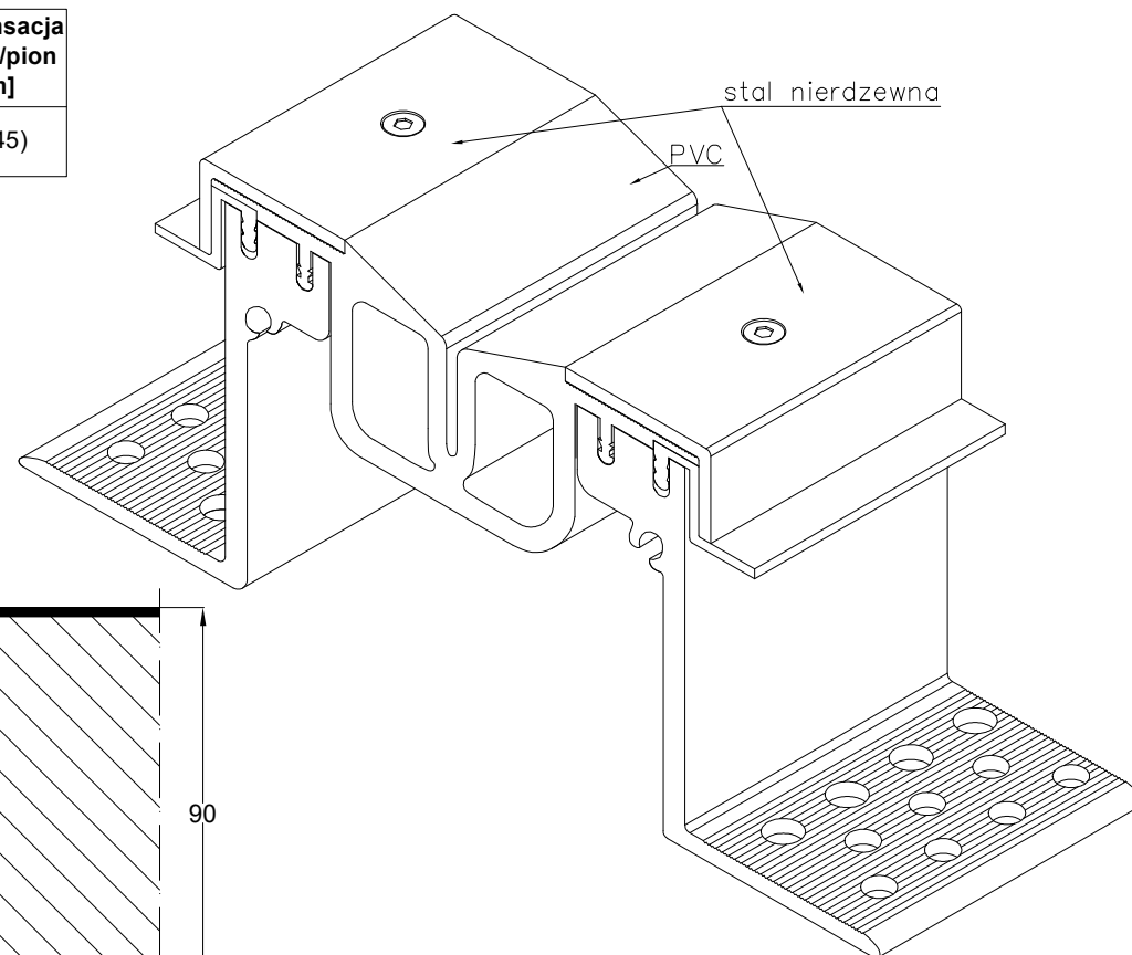
PROFIL DYLATACJNY GA 88.45.90 S RZUT AKSONOMETRYCZNY
