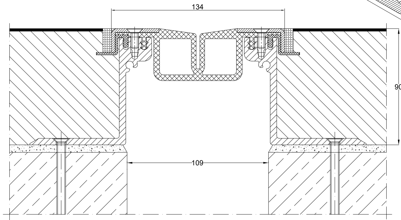
PROFIL DYLATACJNY GA 88.45.90 S PRZEKRÓJ
