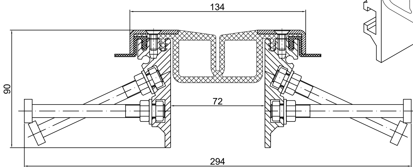
CONECTO GA 88.45.90& S PRZEKRÓJ
