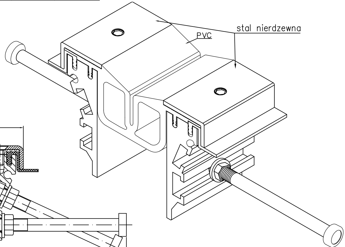
CONECTO GA 88.45.90& S RZUT AKSONOMETRYCZNY
