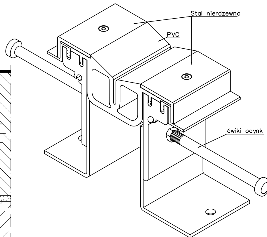
CONECTO PARK GA 88.45.120& S z ocynkowanymi ćwikami RZUT AKSONOMETRYCZNY
