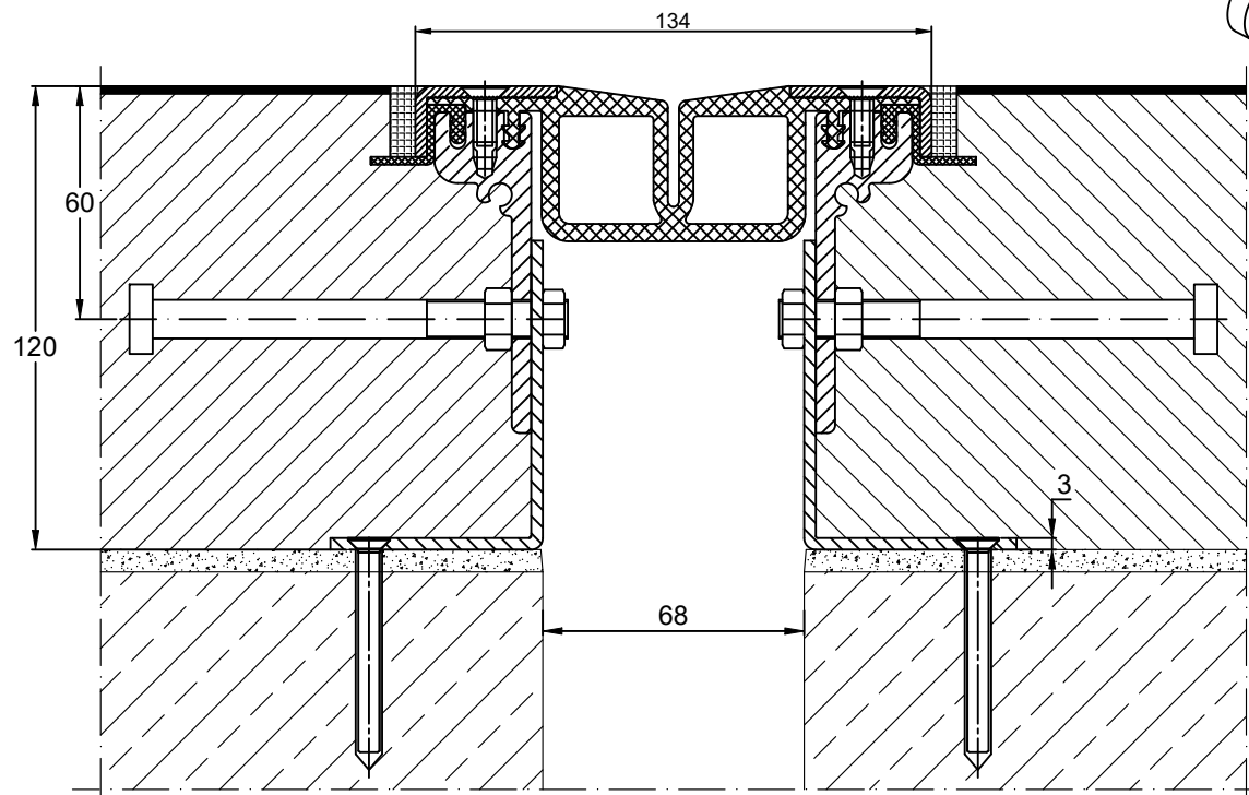
CONECTO PARK GA 88.45.120& S z ocynkowanymi ćwikami PRZEKRÓJ
