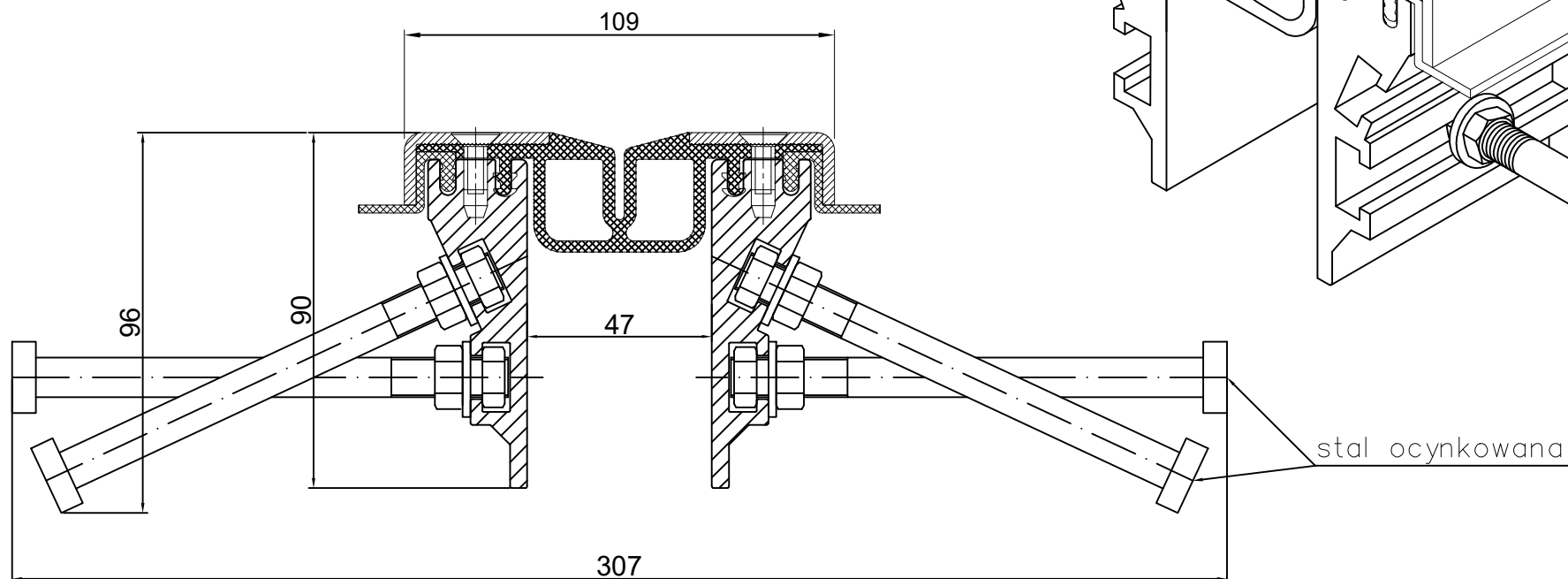
CONECTO GA 63.30.90& S PRZEKRÓJ
