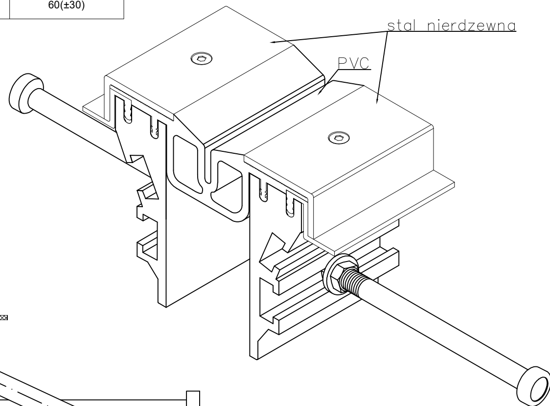
CONECTO GA 63.30.90& S RZUT AKSONOMETRYCZNY
