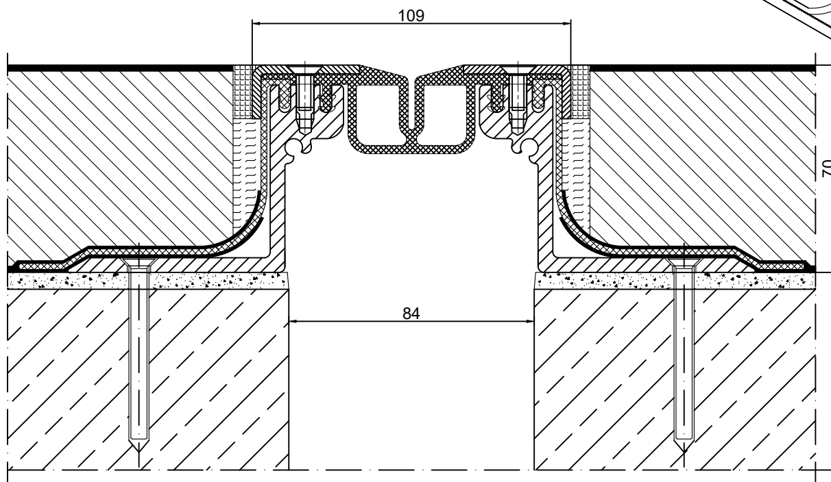
CONECTO GA 63.30.70L PRZEKRÓJ
