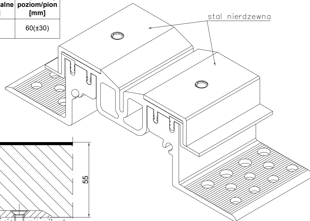
CONECTO GA 63.30.55 S RZUT AKSONOMETRYCZNY
