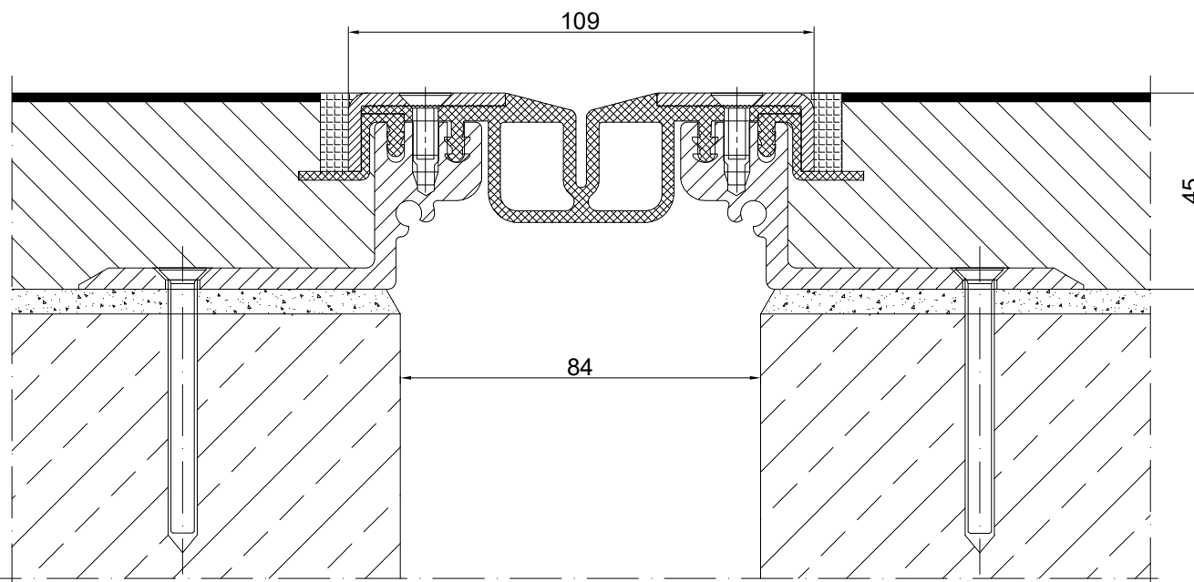
PROFIL DYLATACJNY GA 63.30.45 S PRZEKRÓJ
