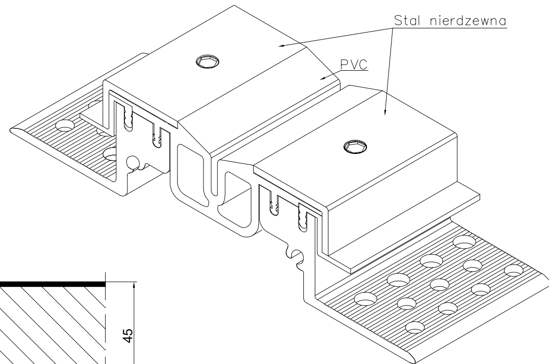
PROFIL DYLATACJNY GA 63.30.45 S RZUT AKSONOMETRYCZNY
