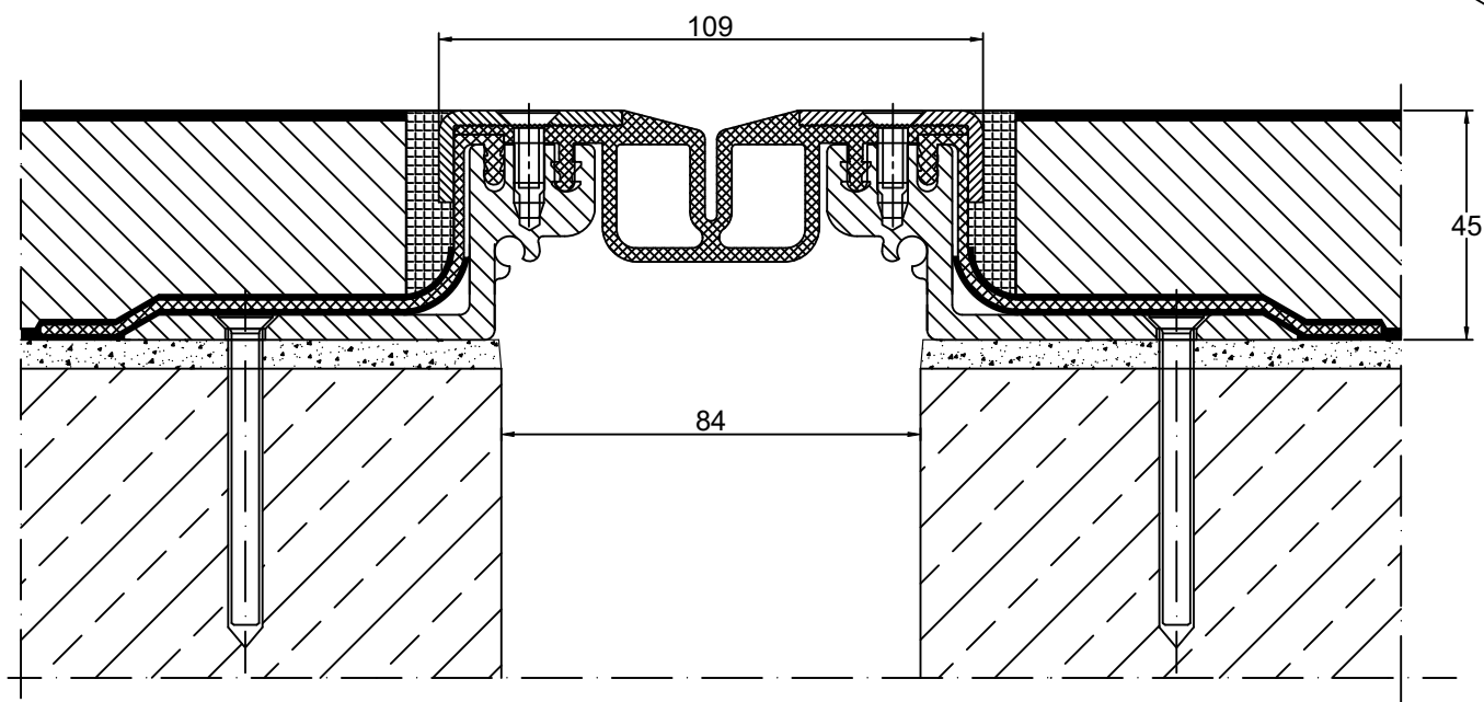
PROFIL DYLATACYJNY GA 63.30.45 S PRZEKRÓJ
