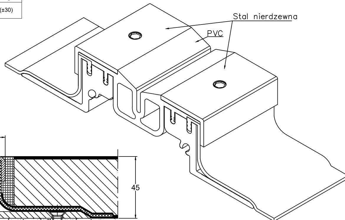
PROFIL DYLATACYJNY GA 63.30.45 S PRZEKRÓJ
