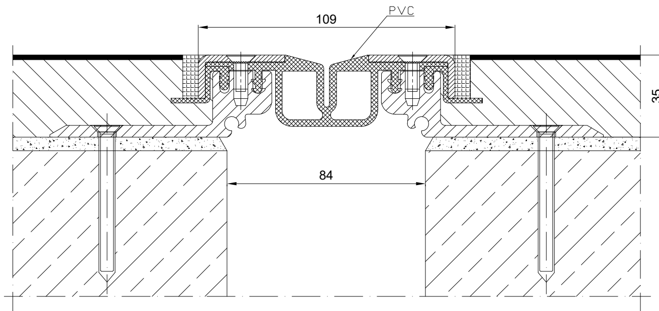
PROFIL DYLATACJNY GA 63.30.35 S PRZEKRÓJ
