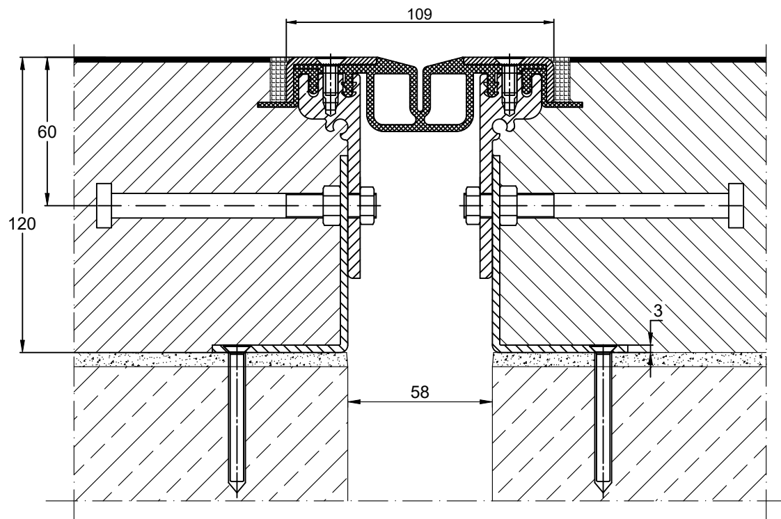
CONECTO PARK GA 63.30.120& S z ocynkowanymi ćwikami PRZEKRÓJ
